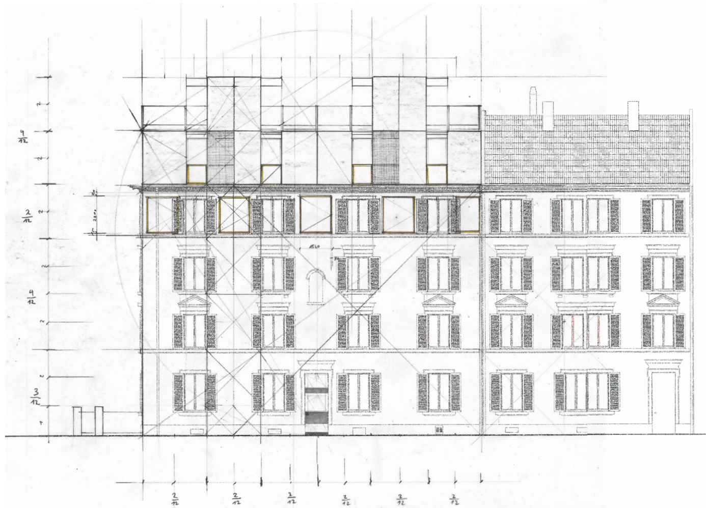
Strassenfassade (Nordosten) 0 1 2 5 10 m
