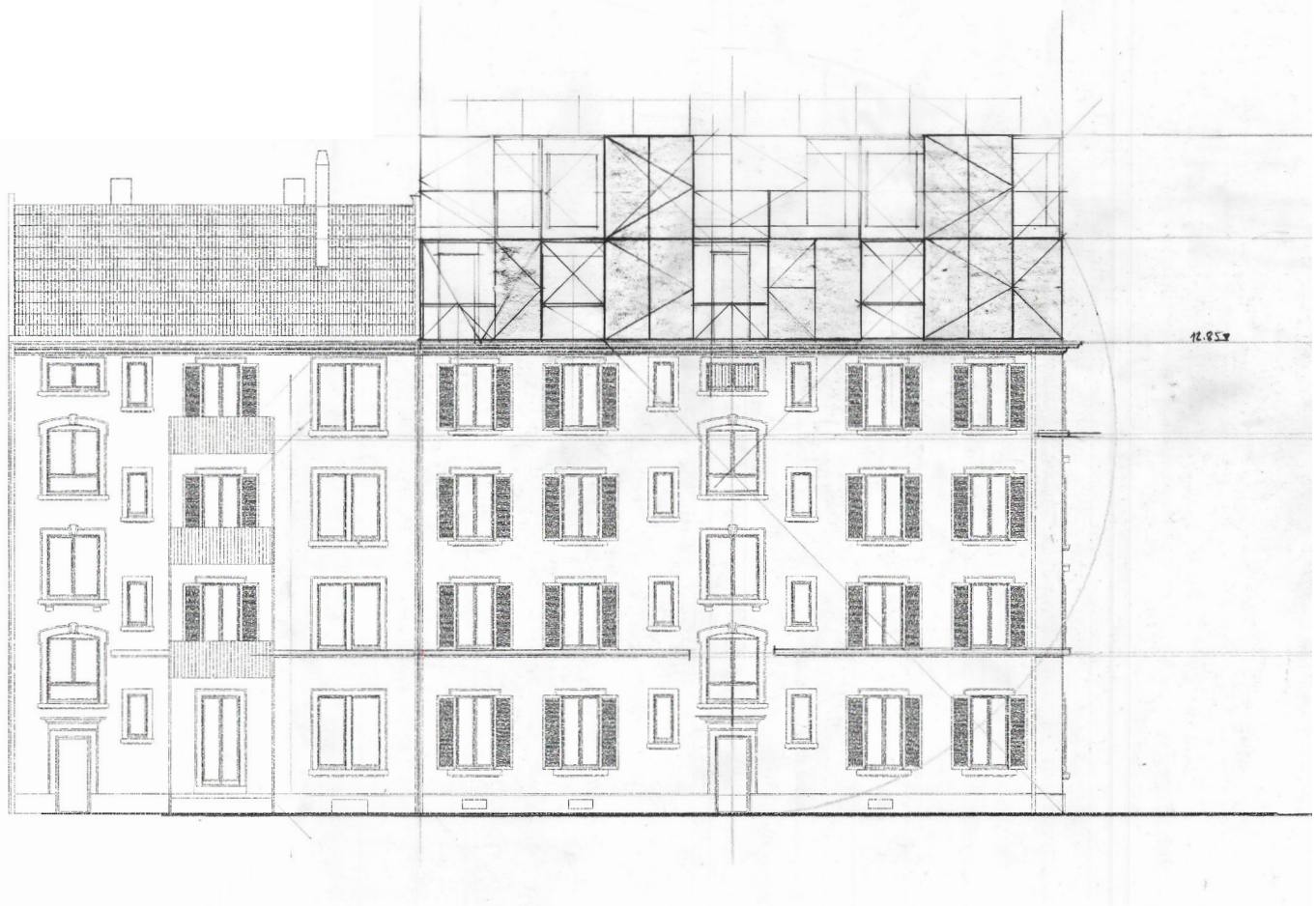
Hoffassade (Südwesten) 0 1 2 5 10 m
